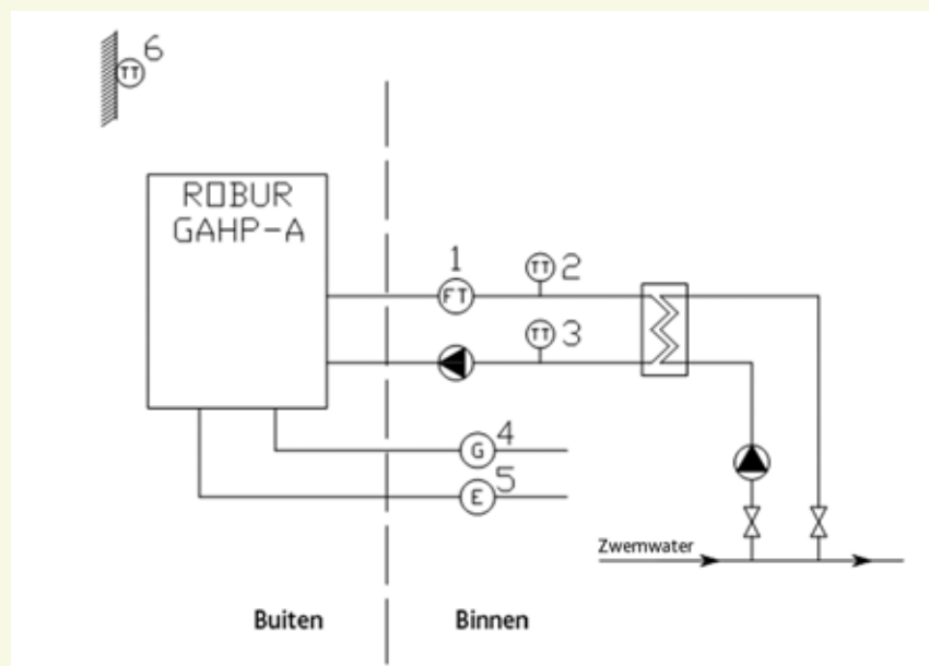
-Figuur 2- Hydraulische inpassing luchtgekoelde gasabsorptiewarmtepomp
