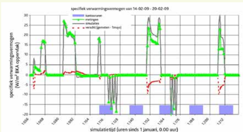
-Figuur 1- Casestudy: specifiek verwarmingsvermogen; gemeten en berekende waarden
