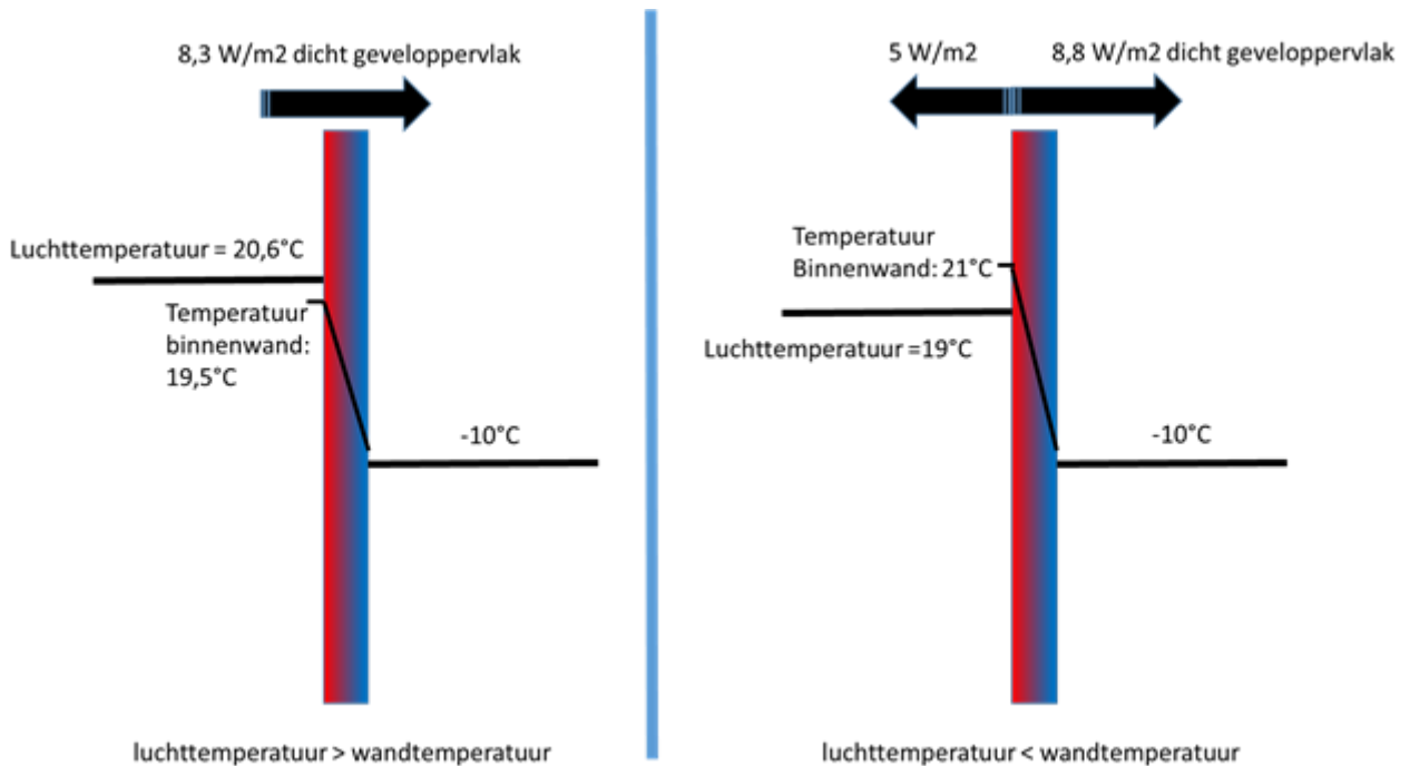
Figuur 2 Hogere wandtemperaturen leiden tot extra vermogensverlies aan de buitengevel (voorbeeld Rc-waarde = 3,5 \text{ m}^2 \cdot \text{K/W} , operationele temperatuur = 20^\circ\text{C} , buitentemperatuur = -10^\circ\text{C} ).
